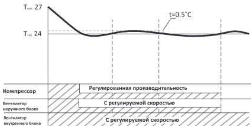
Рис.2 Режим охлаждения инверторной технологии ( \pm 0,5^{\circ}\text{C} )
